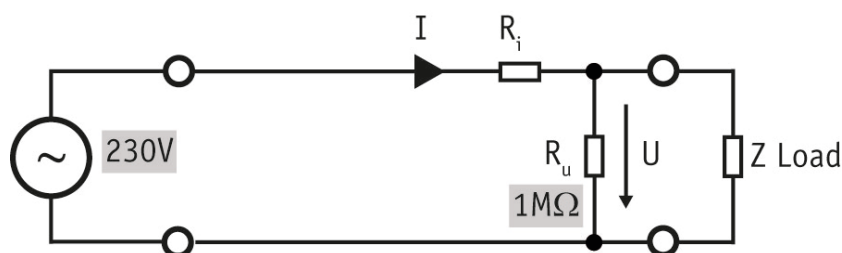
Abb. 1: Spannungsrichtige Messung.
