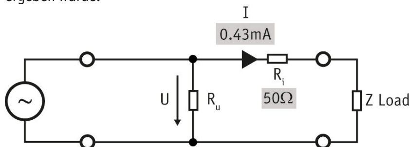
Abb. 2: Stromrichtige Messung. Bevorzugt, wenn der Spannungsabfall über R_i sehr gering ist im Verhältnis zum Spannungsabfall über den Verbraucher Z. Verlustleistung in R_i : 9,2 \mu W
